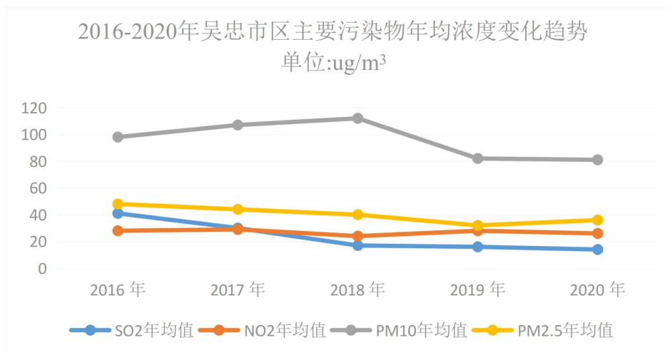
2016-2020年吴忠市区主要污染物年均浓度变化趋势 (单位: μg/m 3 )
